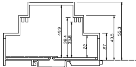
BARRA DIN
