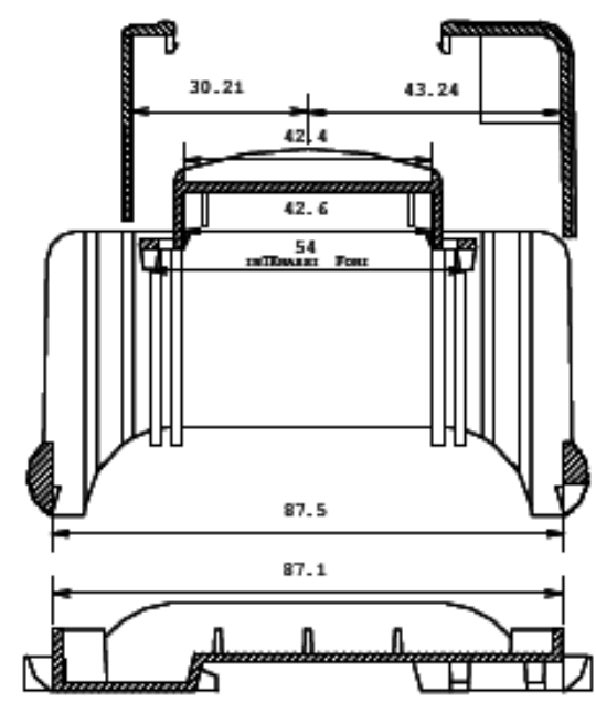
Sez. A-A
