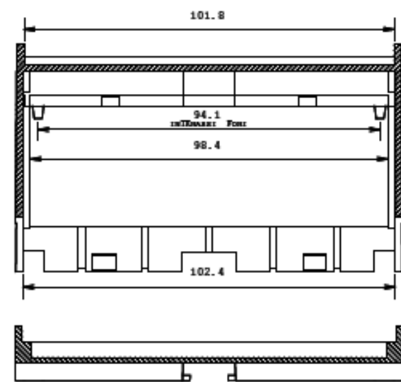
Sez. B-B
