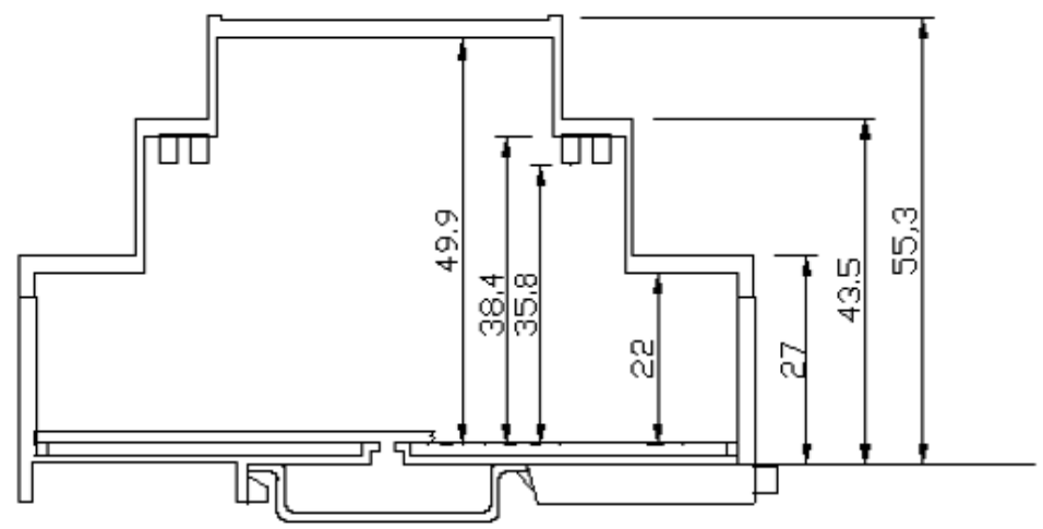
BARRA DIN
