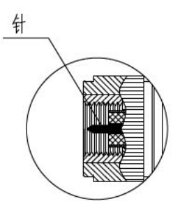
ViewA: 2:1
