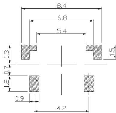
P.C.B LAND DIMENSION
